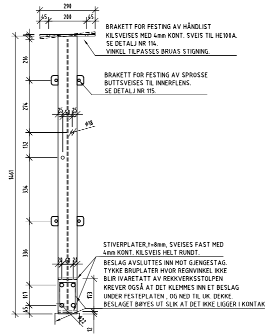
OPPRISS REKKVERKSSTOLPE PÅ DEKKET
