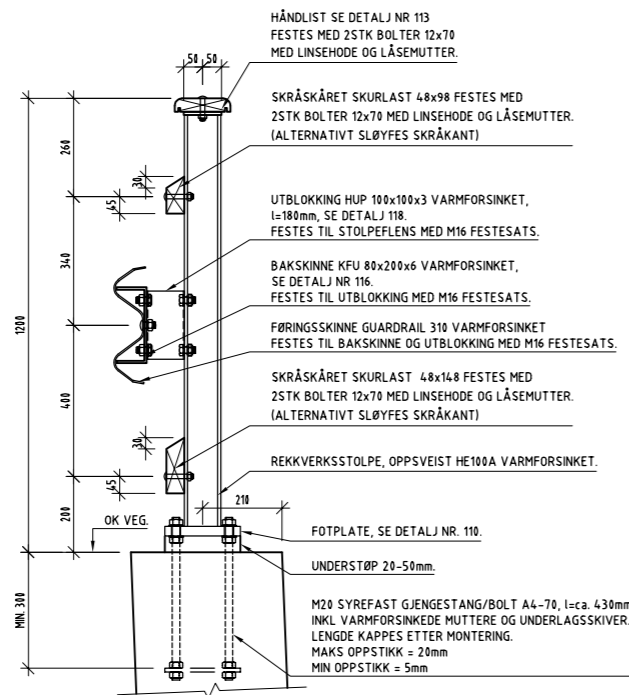
REKKVERKSSTOLPE PÅ LANDKAR
