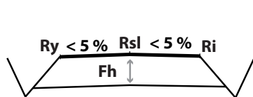
Figur 4.6 Tøssidig tøverrfall
