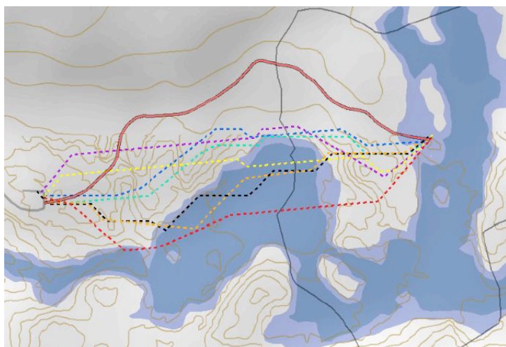
Figur 3. En sammenligning av beregnede traséforslag for driftsveier (stiplet), med og uten markfuktighetsinformasjon. Rød heltrukken er den faktiske driftsveien.
