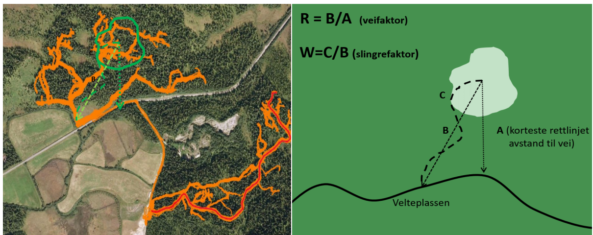
Figur 12. Bruk av lassbærerens sporlogg data (venstre) til beregning av driftsveiens geometri (høyre).
