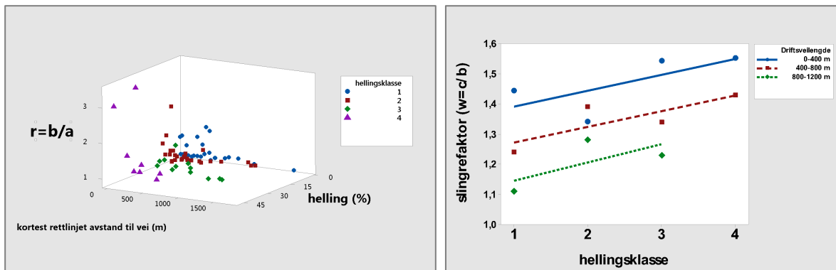
Figur 13. Effekten av avstand fra vei og terreghelling på driftsveiens geometri (veifaktor= r på venstre, slingrefaktor= w til høyre). Kortest rettlinjert avstand til vei.
